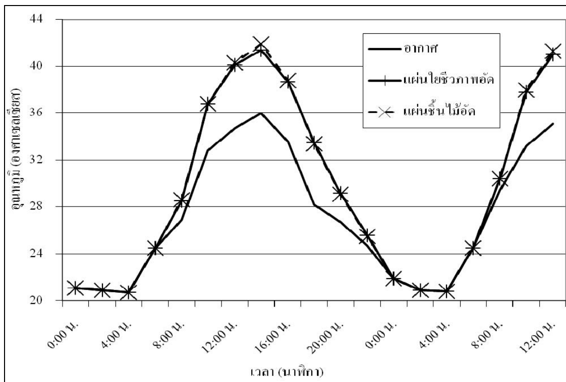
รูปที่ 4.14 อุณหภูมิภายในอาคารจำลองที่ผนังด้านในมีการติดตั้งแผ่นใยชีวภาพอัดความหนาแน่นปานกลางที่ผสมเส้นใยอัตราส่วน CC50 และแผ่นฉนวนไม้อัดชนิดอัดราบทั่วไป
