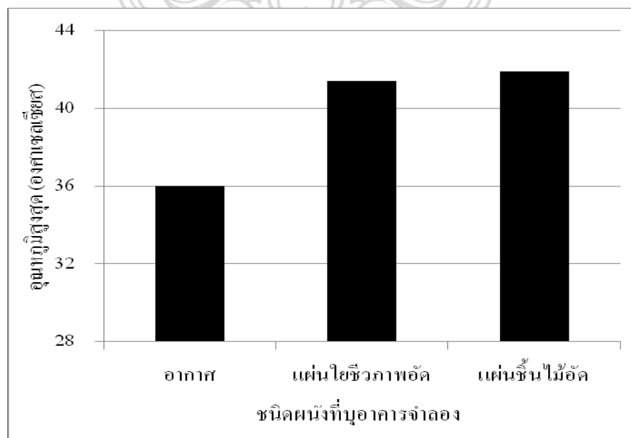
รูปที่ 4.15 อุณหภูมิสูงสุดในอาคารจำลองที่ผนังด้านในมีการติดตั้งแผ่นใยชีวภาพอัดความหนาแน่นปานกลางที่ผสมเส้นใยอัตราส่วน CC50 และแผ่นฉนวนไม้อัดชนิดอัดราบทั่วไป
